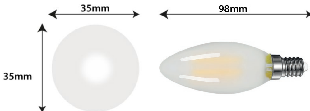
Dimensioni Dimensions
